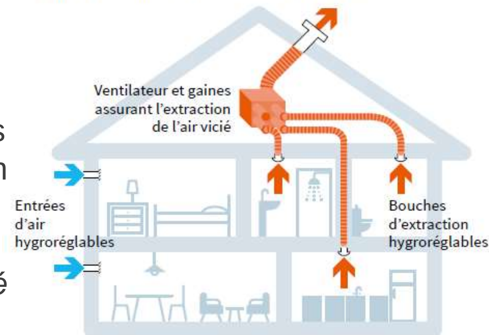
PRINCIPE DE LA VMC SIMPLE FLUX HYGRORÉGLABLE
